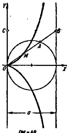
23. Циссоида Дюклена
