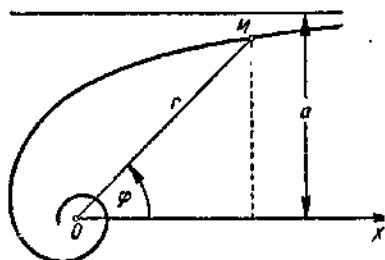
31. Гиперболическая спираль r = \frac{a}{\varphi} ( r > 0 ).
