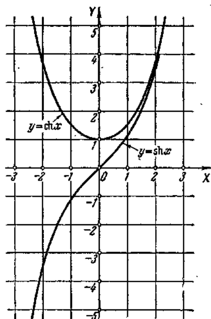
17. Графики гиперболических функций
