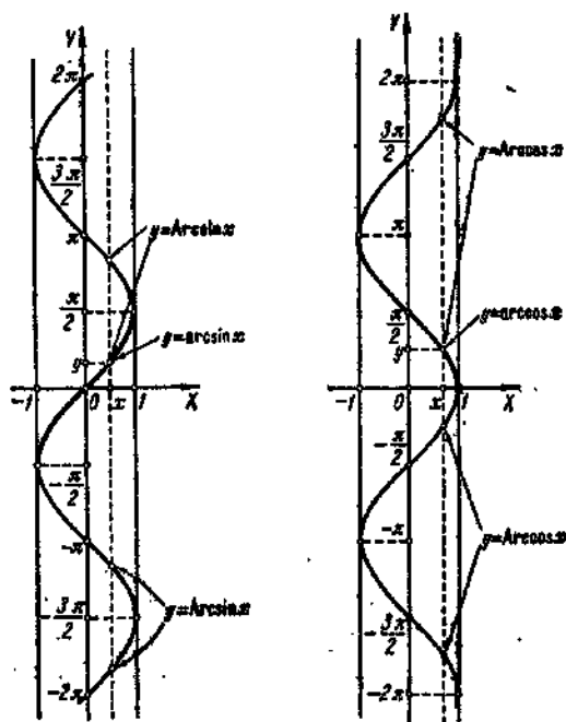
12. Графики обратных тригонометрических функций y = \operatorname{Arcsin} x и y = \operatorname{Arccos} x .
