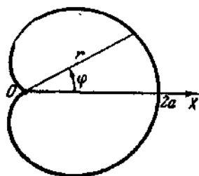
28. Кардиоида
