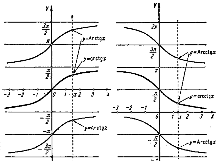
13. Графики обратных тригонометрических функций y = \text{Arctg} x и y = \text{Arcctg} x .
