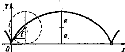
26. Циклоида
