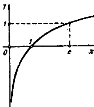
15. Логарифмическая кривая y = \ln x .
