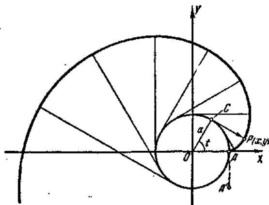
29. Эвольвента (развертка) окружности
