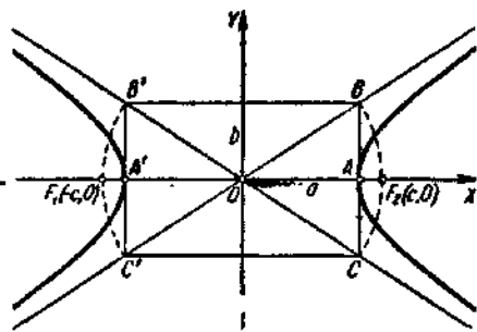
20. Гипербола
