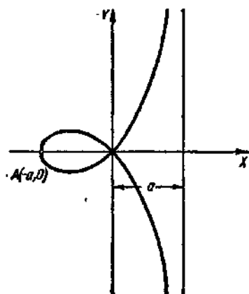
24. Строфонда
