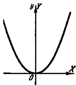
1. Парабола y = x^2 .
