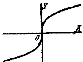
7. Кубическая парабола y = \sqrt[3]{x} .
