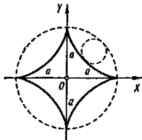
27. Гипоциклода (астроида)
