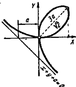
22. Декартов лист x^3 + y^3 - 3axy = 0 или
