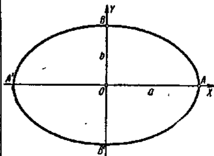
19. Эллипс
