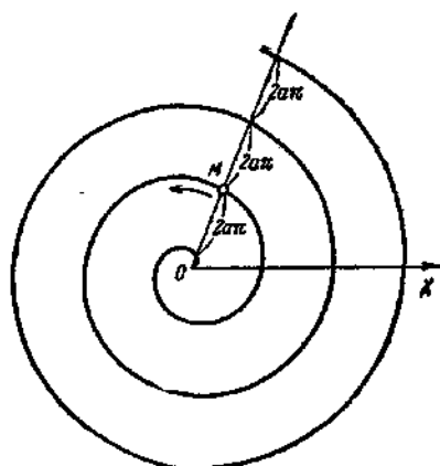
30. Спираль Архимеда r = a\varphi ( r \geq 0 ).
