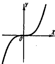
2. Кубическая парабола y = x^3 .
