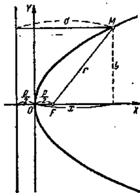
21. Парабола y^2 = 2px .
