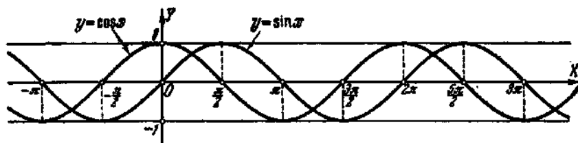
9. Синусоида и косинусоида y = \sin x и y = \cos x .
