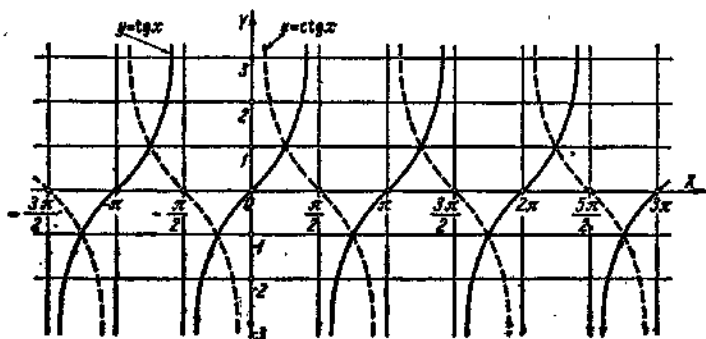
10. Тангенсоида и котангенсоида y = \tan x и y = \cot x .
