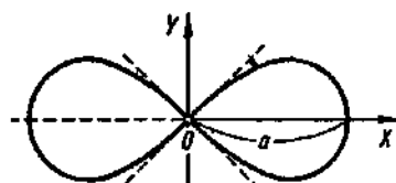
25. Лемниската Бернулли
